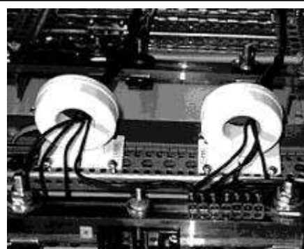
Bild 2.1.4 Montering av summaströmtransformatorer
