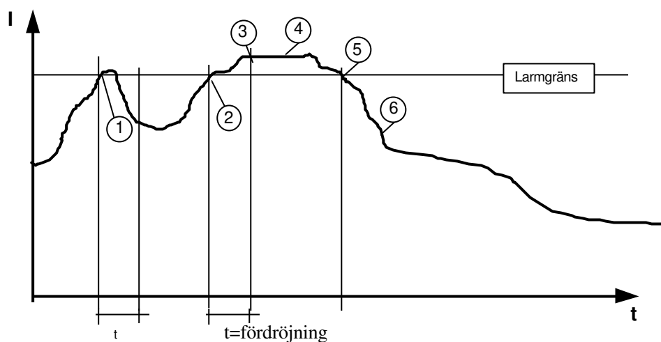
Bild 4.2.1 Hur strömlarm uppkommer och deaktiveras
