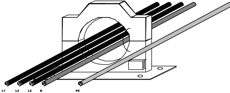
Bild 2.3.1 Kabeldragning genom summaströmtransformatorn.
