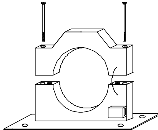
Bild 2.3.4 Summaströmtransformator VMI(K)-200
